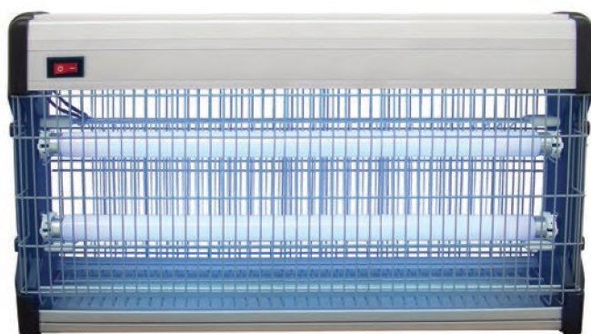
Уничтожитель насекомых GASTRORAG / EGO-02-40W Инсектицидная лампа, УФ, настенная, площадь действия 150 кв.м, материал корпуса – алюминий Габариты (дл.х ш.х в.): 668x102x320 мм Мощность: 0,04 кВт
